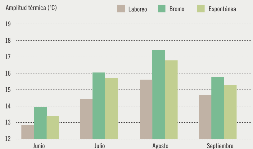
Gráfico 2. Amplitud térmica
